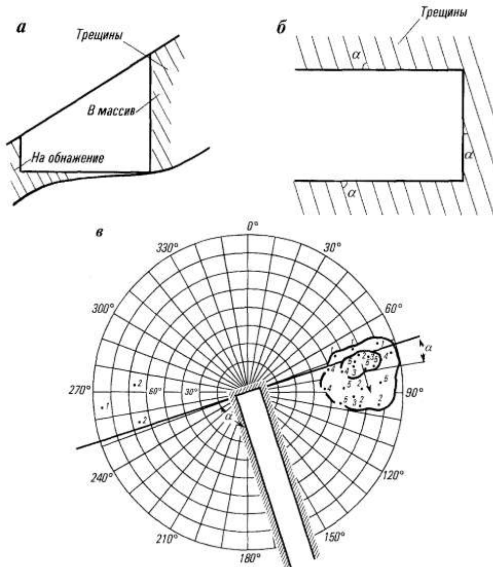
Рис. 11. Ориентировка трещин относительно обнажения выработки: a — разрез; б — план; в — круговая диаграмма; \alpha — угол встречи трещины с обнажением
