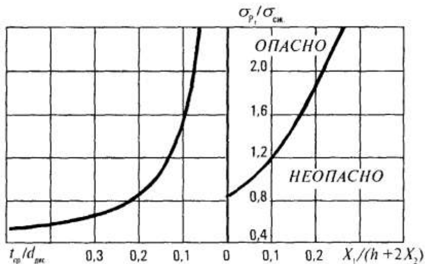
Рис. 9. Номограмма для определения категории удароопасности участков массива по дискованию керна:
