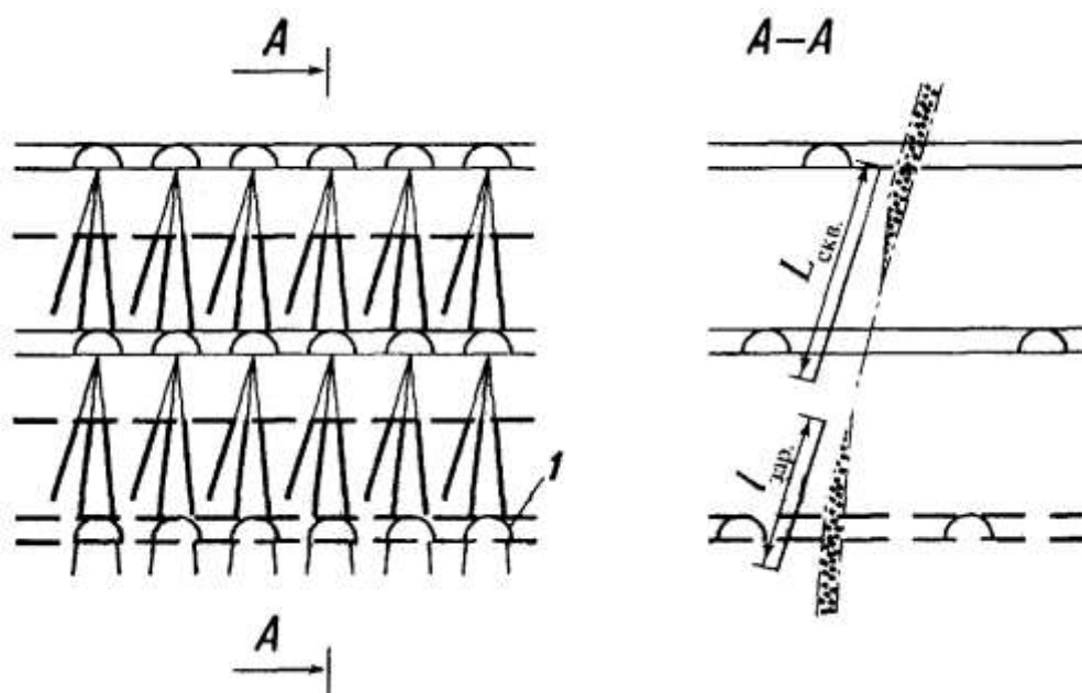
Рис. 4. Схема расположения скважин вблизи тектонического нарушения.
