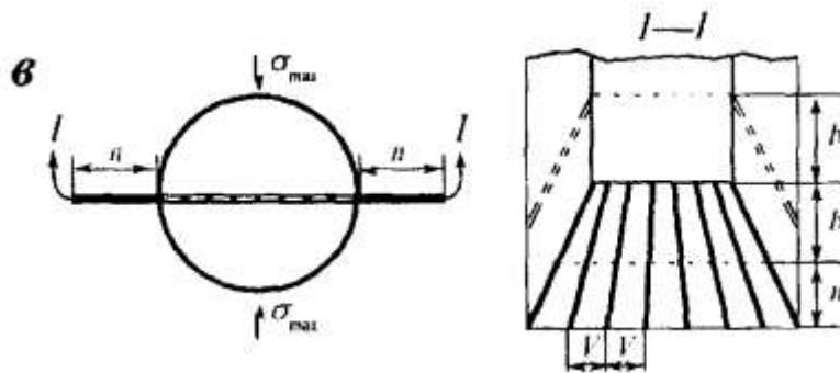
Рис. 1. Схемы камуфлетного взрывания по рядам шпуров:
