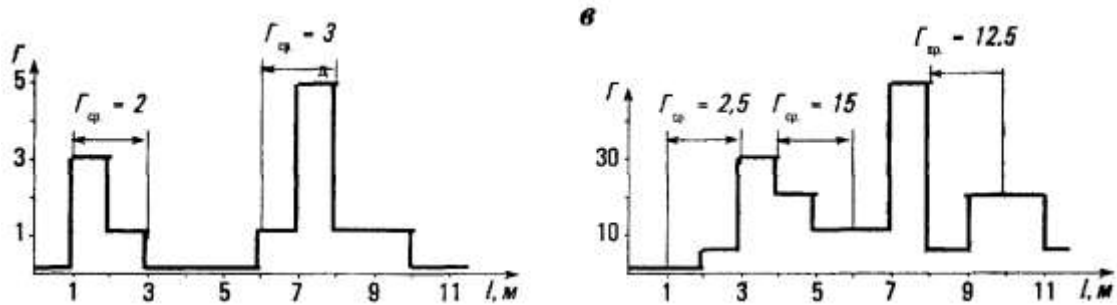
Рис. 10. Определение интенсивности трещин: а — определение плотности (числа) трещин; б, в — примеры оценки средней плотности (числа) \Gamma_{\text{ср}} трещин поперечной направленности по длине участка выработки l
