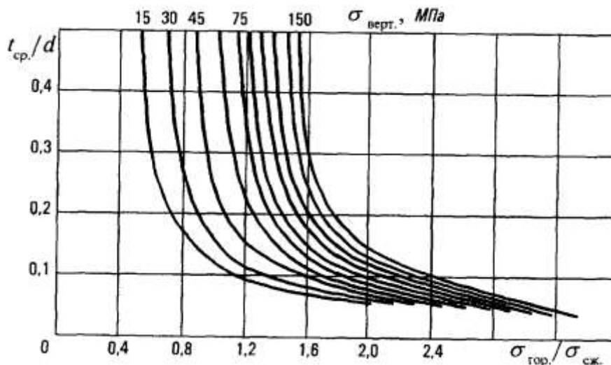
Рис. 12. Номограмма для оценки напряженного состояния пород \sigma_{гор.}/\sigma_{ск.} по дискованию керна по данным бурения геологоразведочных скважин при различных вертикальных напряжениях, определяемых величиной \gamma H :
