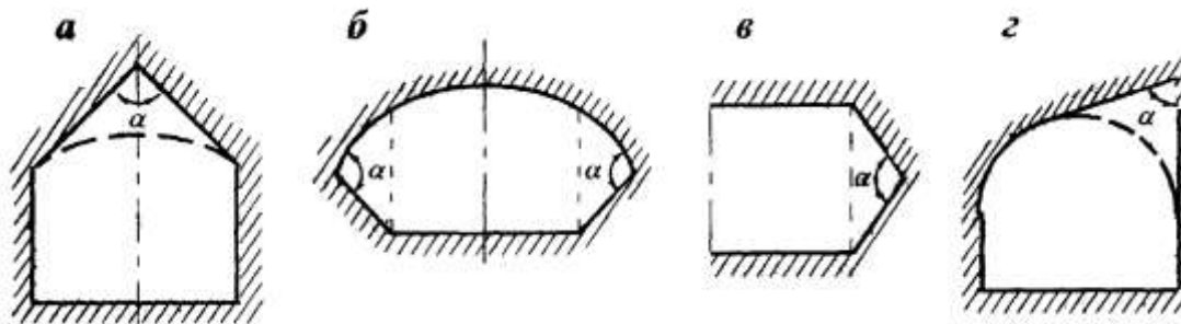
Рис. 5. Полигональная форма выработок при расположении мест разрушения: a — в кровле, б — в стенках, в — в забое, г — в сопряжении кровли со стенкой; \alpha \leq 100^\circ — угол разрушения
