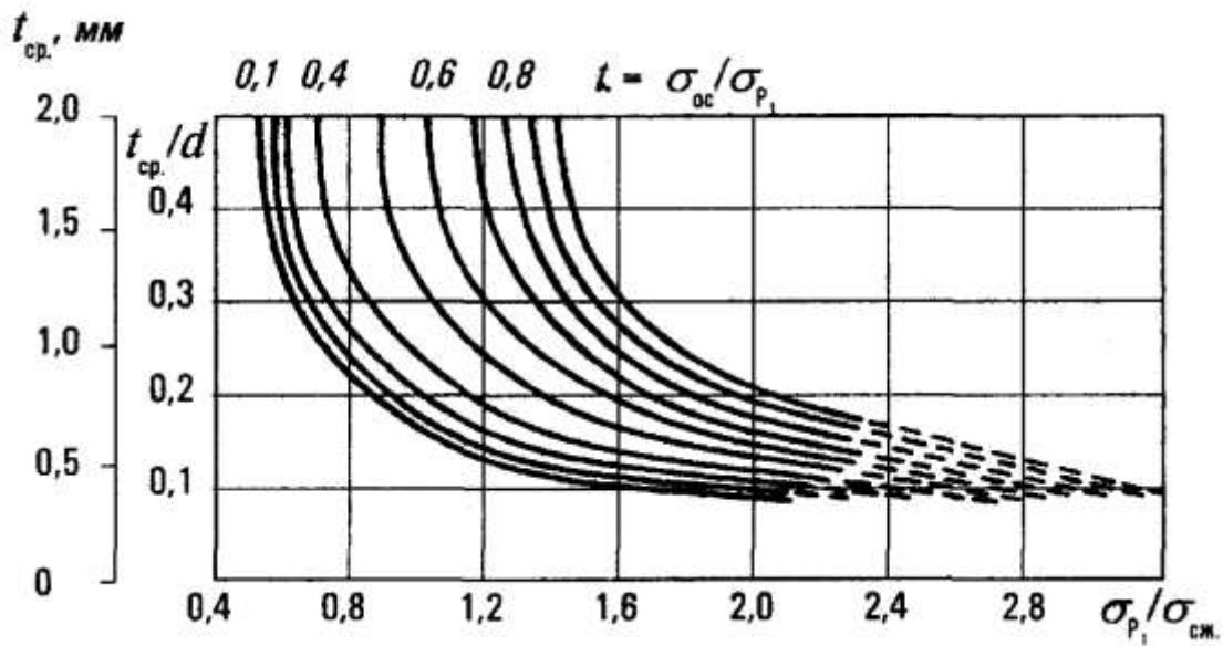
Рис. 6. Зависимости параметров дискования керна t_{cp}/d_{дис} от уровня напряженности массива \sigma_{p_1}/\sigma_{сж.} при различных соотношениях между осевыми и радиальными напряжениями \sigma_{0c}/\sigma_{p_1} :
