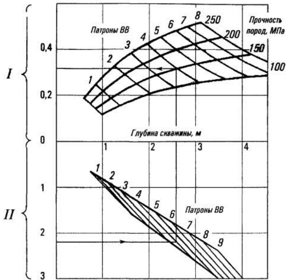
Рис. 2. Номограмма для определения параметров камуфлетного взрыва ряда шпуров (масса патронов ВВ 0,2 кг) I — относительная длина заряжаемой части скважины; II — расстояние до максимума напряжений, м.
