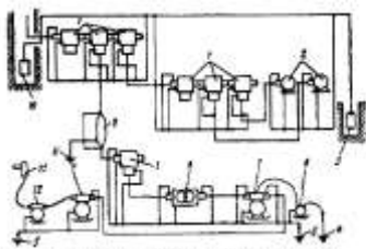
Рис. 1. Принципиальная схема заземляющей сети в шахте: 1 - комплектные распределительные (КРУ); 2 - электродвигатели насосов; 3 - главный заземлитель в водосборнике; 4 - дополнительный заземлитель реле утечки; 5 - местные заземлители; 6 - реле утечки; 7 - автоматический выключатель; 8 - трансформатор; 9 - кабельная муфта; 10 - главный заземлитель в зумпфе; 11 - комбайн; 12 - магнитный пускатель.
