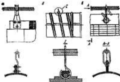
Рис. 21. Примерные схемы заземления металлических деталей гибких вентиляционных труб: а - типа М (прорезиненных); б - типа ТВ (прорезиненных с металлической спиралью); в - типа К (алюминиевых)
