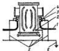
Рис. 9. Схема заземления трансформатора: 1 - броня кабеля; 2 - заземляющий зажим; 3 - катушка; 4 - переключатель; 5 - заземляющие проводники; 6 - местный заземнитель.
