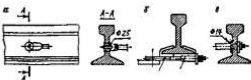
Рис. 12. Схема присоединения заземляющего проводника к рельсу: а - пулькой; б - башмаком; в - медной шайбой и гайкой
