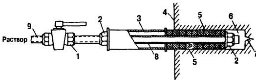
Рис. 1 Установка иньектора в скважине:
