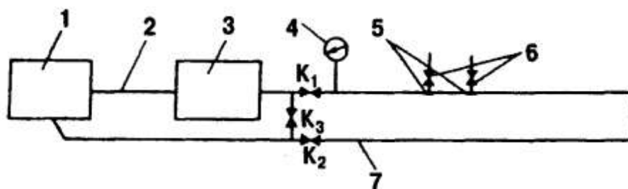
Рис. 2. Принципиальная схема нагнетания цементного раствора:
